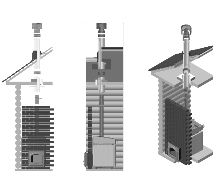
Рис. 10. Схема установки печи
