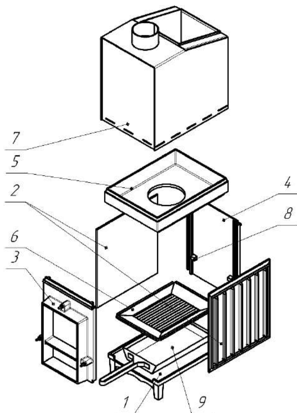
Рис.13 Схема сборки топочного агрегата печи Сударушка Семейная РК в облицовке из природного камня с фасками, Сударушка Семейная РК в облицовке из природного камня без фасок.
