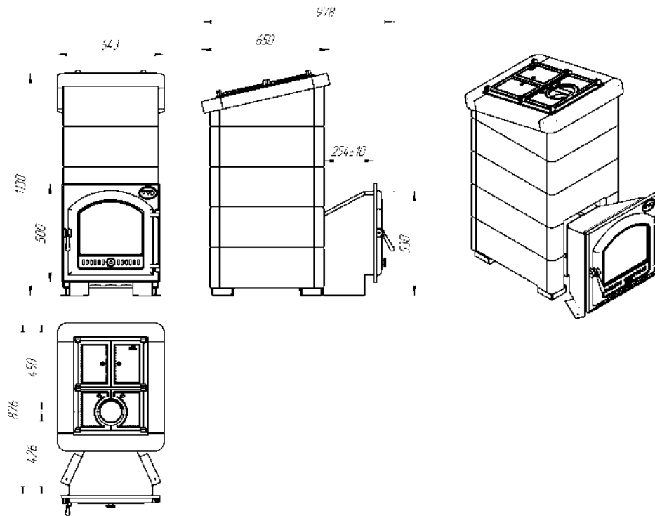
Рис. 4 Сударушка Семейная РК в облицовке из природного камня без фасок
