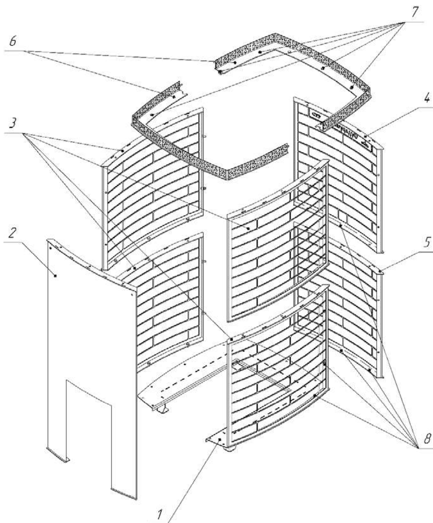
Рис.19 Схема сборки декоративно защитного ограждения печи Сударушка Чистопар
