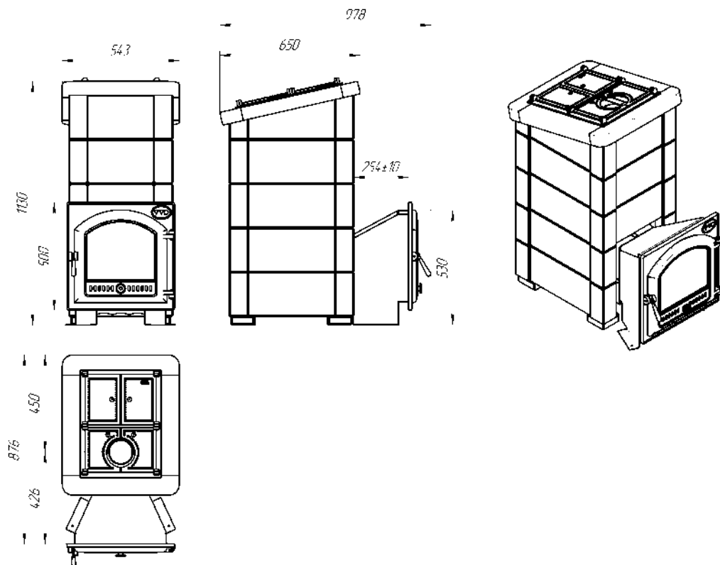
Рис.3 Сударушка Семейная РК в облицовке из природного камня с фасками
