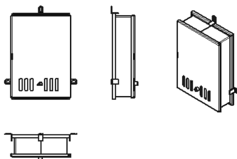
Рис. 7 Короткий топочный тоннель КТК из нержавеющей стали.
