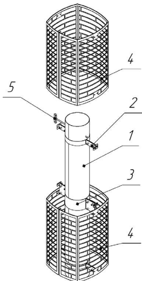
Рис.20 Схема сборки декоративно защитного ограждения печи Сударушка Чистопар
