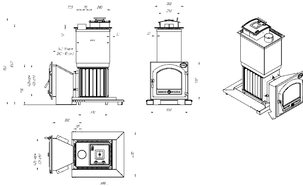
Рис. 6 Топочный агрегат для бани Сударушка Семейная
