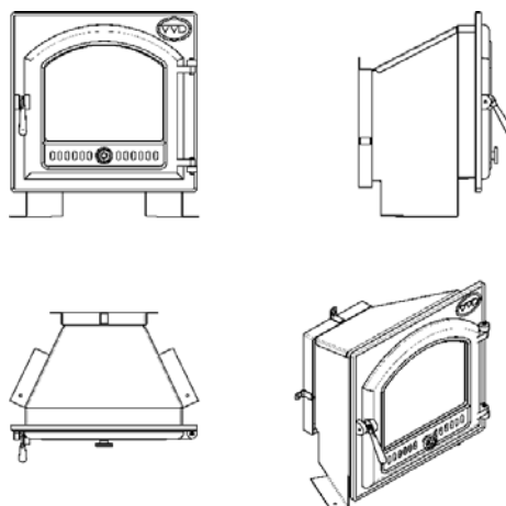
Рис. 9 Тоннель из нержавеющей стали с чугунной дверью со стеклом.
