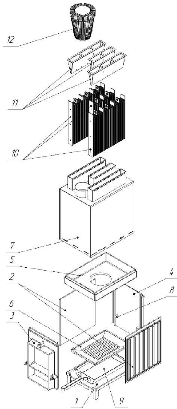
Рис. 14 Схема сборки топочного агрегата печи Сударушка Чистопар.
