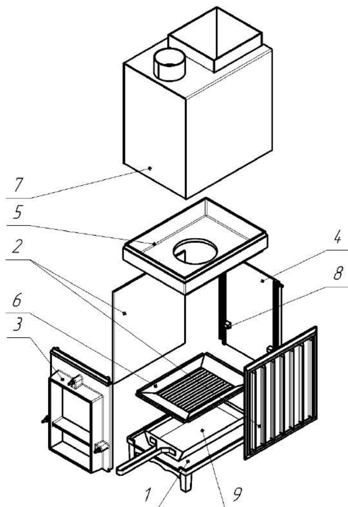
Рис.12 Схема сборки топочного агрегата печи Сударушка Руса-Семейная, Сударушка Семейная.
