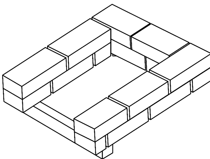
Рис.22 Схема укладки керамического кирпича
