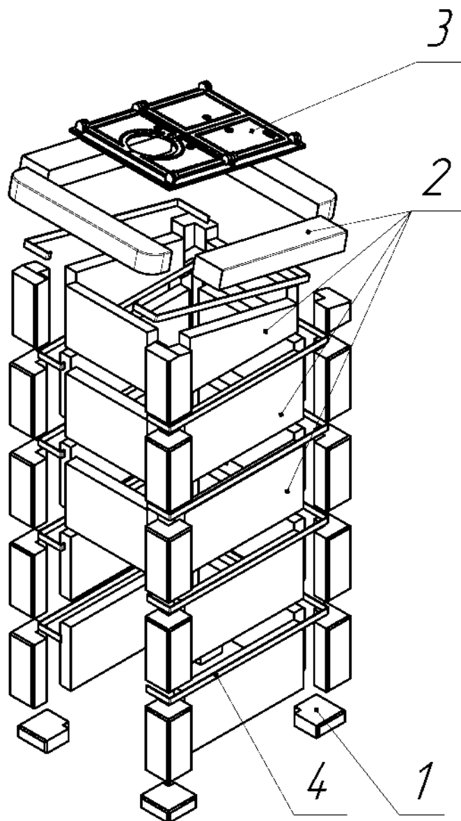
Рис.17 Декоративно-защитное ограждение печи Сударушка Семейная РК в облицовке из природного камня с фасками.
