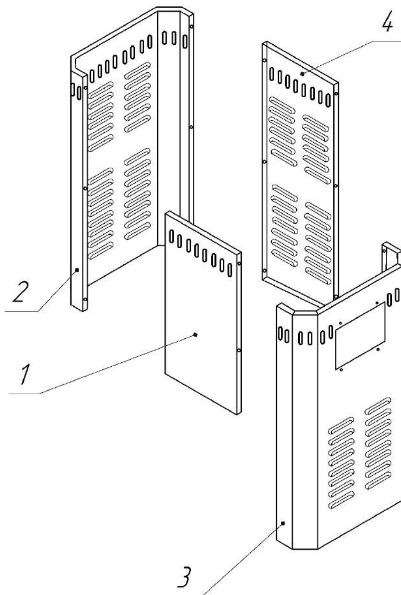
Рис.15 Декоративно-защитное ограждение печи Сударушка М.
